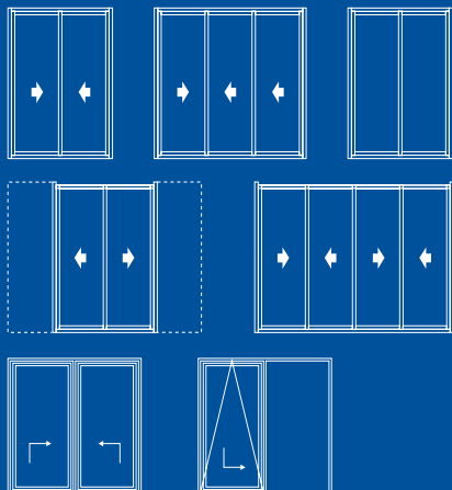
Les ouvertures de baies
